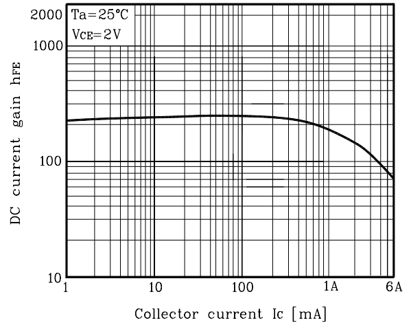
Fig. 2 h_{FE} - I_C
