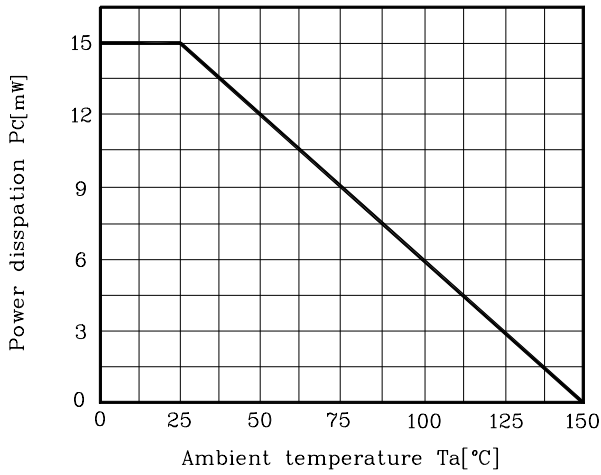
Fig. 1 P_c - T_a
